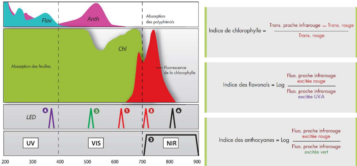
Figure 18 : Principe de mesure des pigments photosynthétiques par le Dualex d'après la plaquette d'utilisation.
